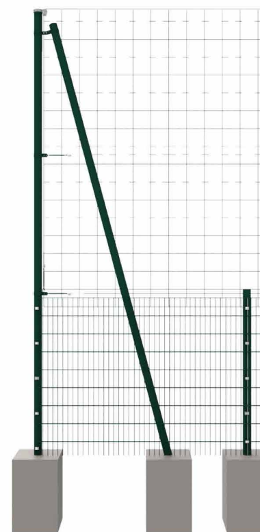
Type 3 : Treillis soudé
