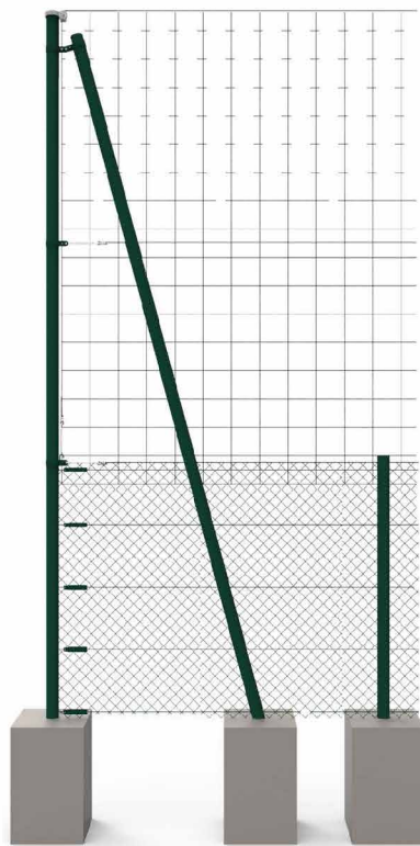
Type 2 : Grillage simple torsion
